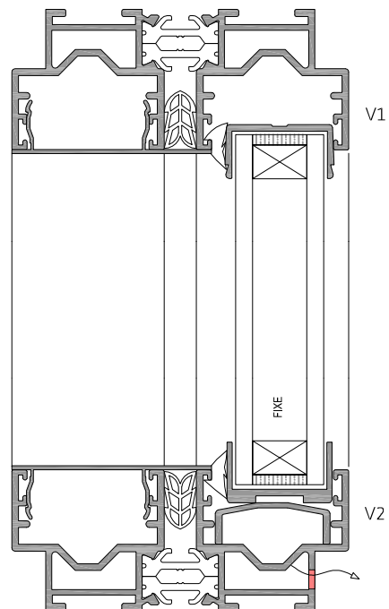
VITRAGE FIXE
